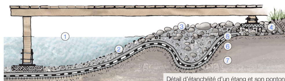
Détail d'étanchéité d'un étang et son ponton
